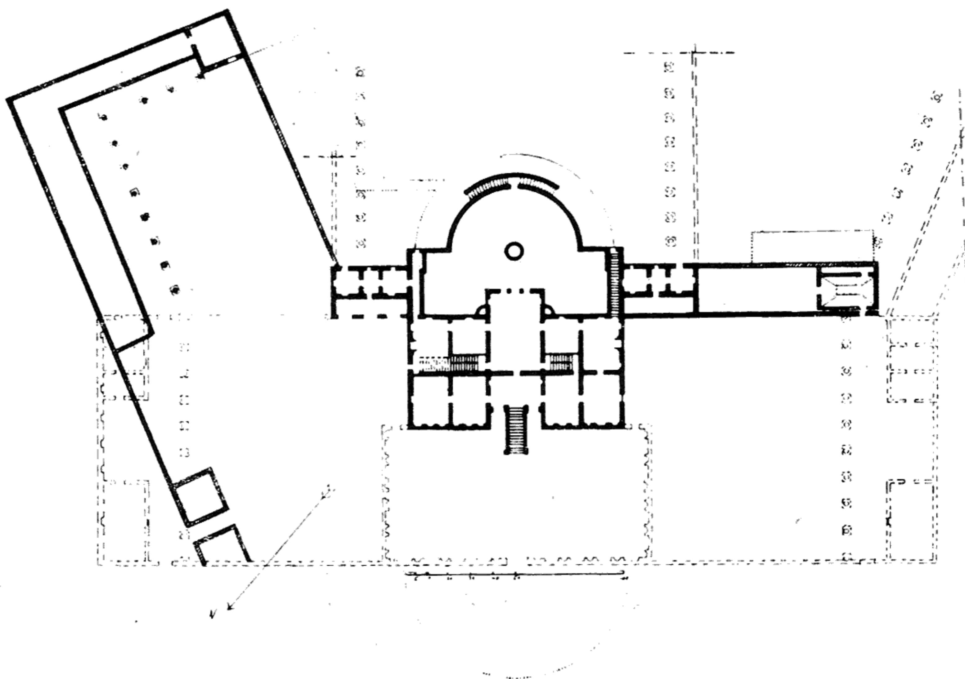
Fig. 5 Planimetria della Villa Godi di Lonedo (secondo la pianta e l'esecuzione).
